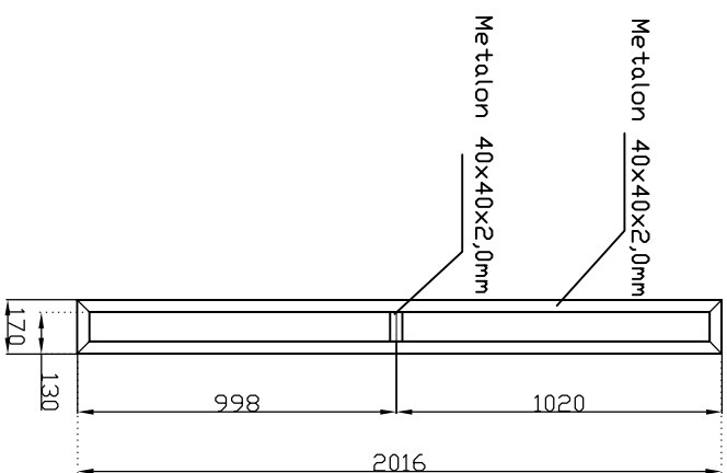
VISTA LATERAL
